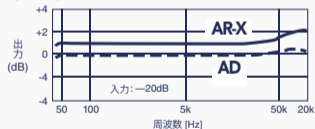
周波数特性
